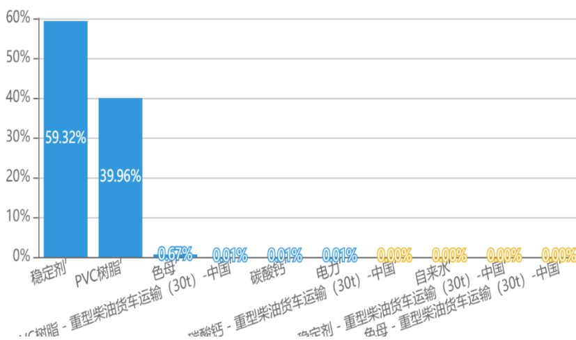
图 6-7 HT 累积贡献
