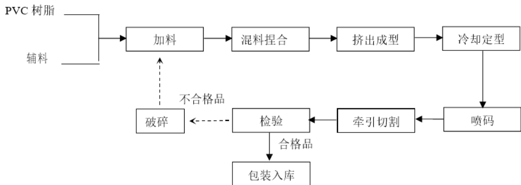
图 2-1 建筑排水用 PVC-U 管材社会年国产工艺流程图
