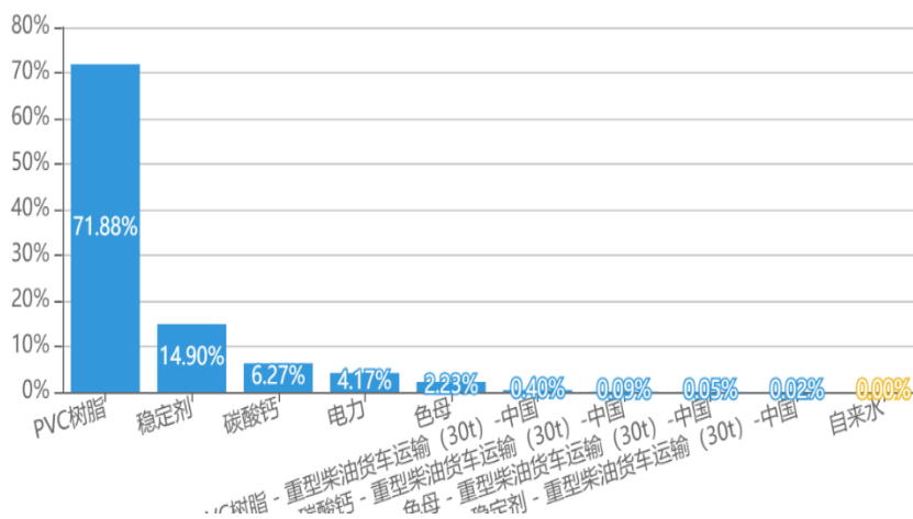
图 6-6 GWP 累积贡献
