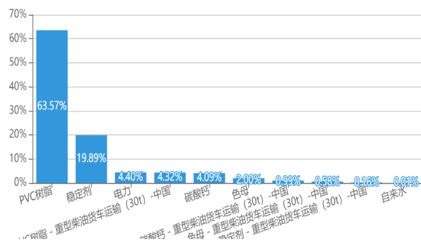
图 6-4 EP 累积贡献
